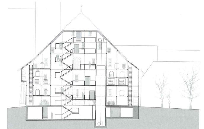
Querschnitt neue Fassadenschicht
