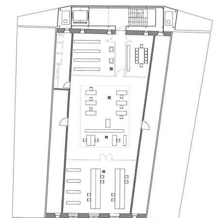
4. Obergeschoss
