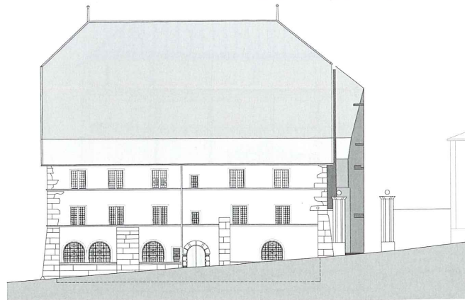
Ostfassade
