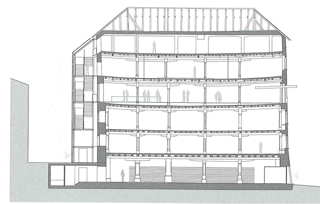
Längsschnitt
