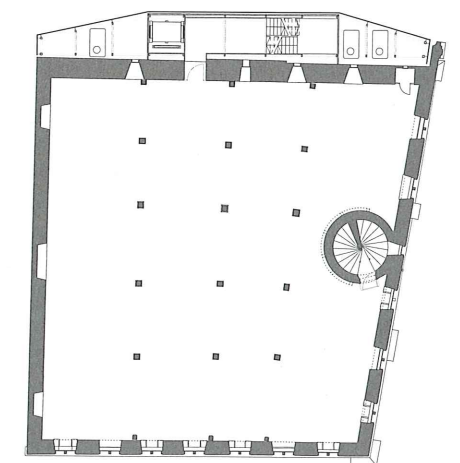
1. Obergeschoss
