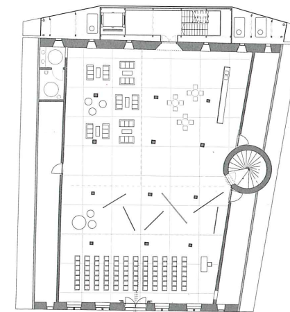
3. Obergeschoss
